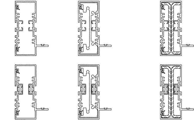
JAMB 'J1'
